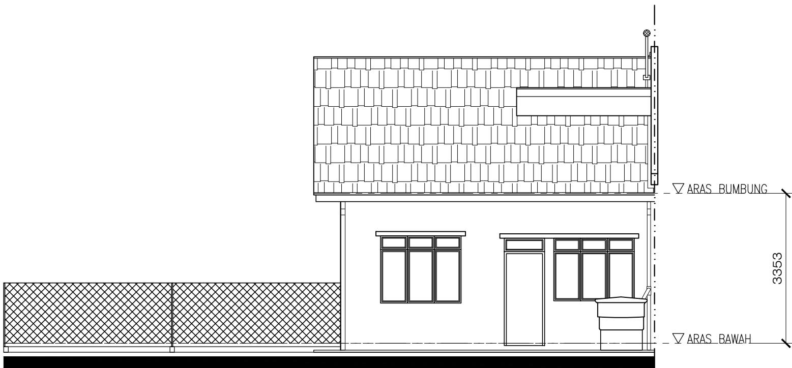
PANDANGAN BELAKANG
