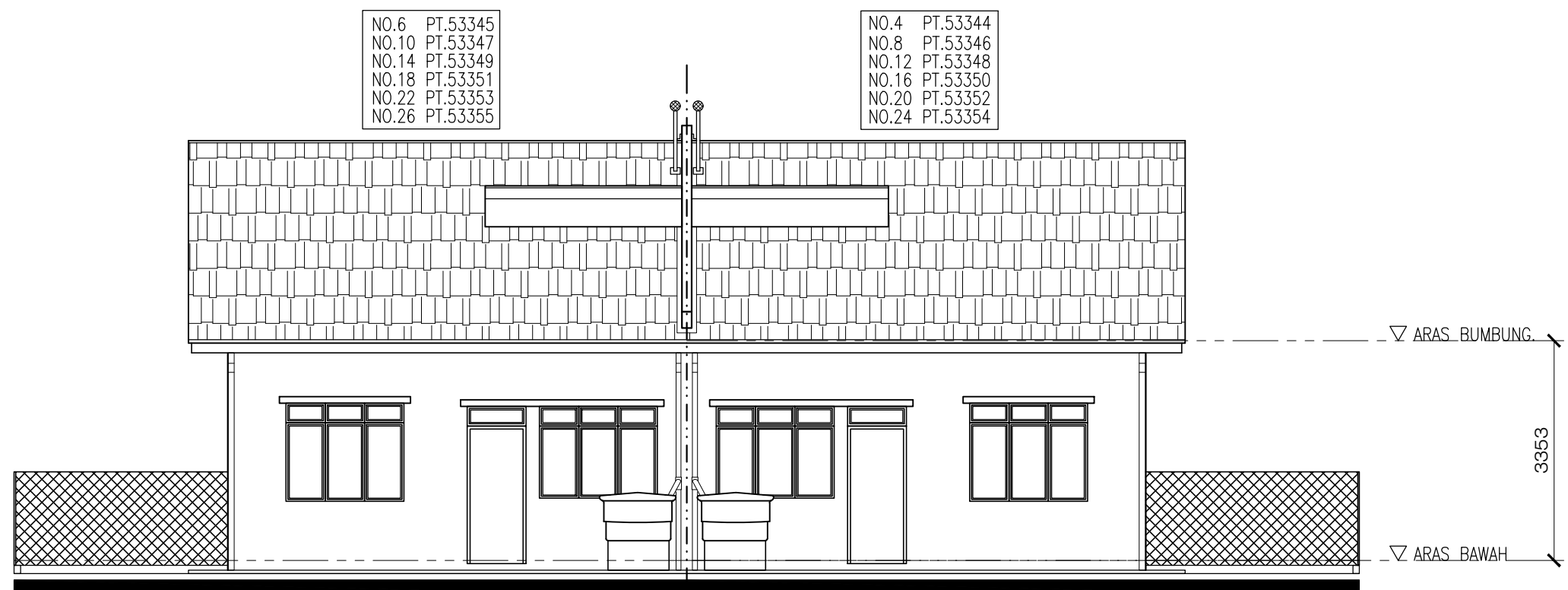
PANDANGAN BELAKANG
